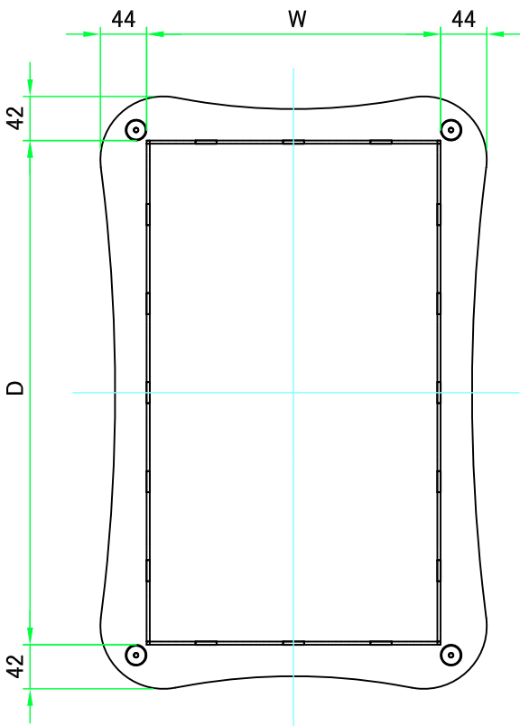
Wパネル1 / W panel 1
