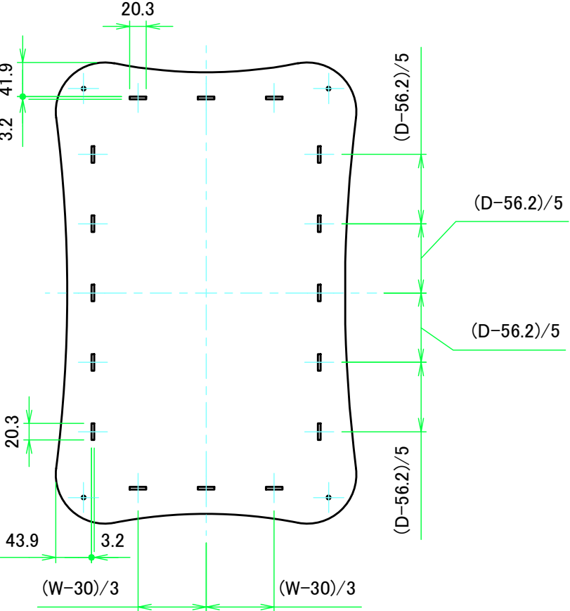
上カバー裏面 / Top cover Backside
