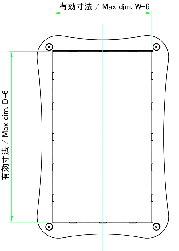
下カバー / Bottom cover
